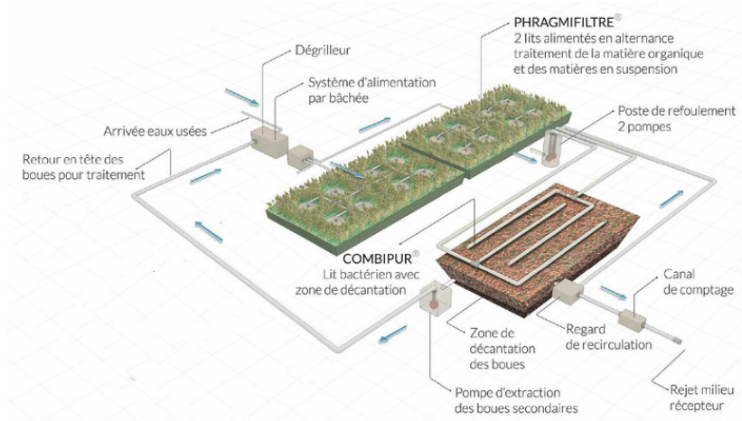
Schéma: Syntea, système Combipur © de Epur Nature
